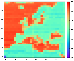
Σχήμα: WRF: Ποσοστό του συνολικού χρόνου που καταναλώνεται σε MPI κλήσεις.
