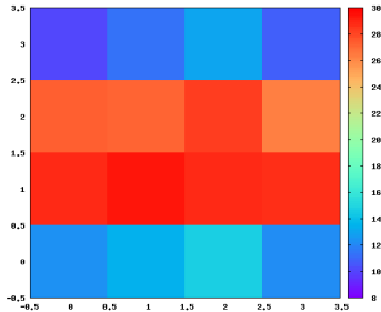
Σχήμα: Load imbalance : Global, 16 cores
