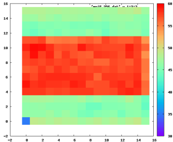
Σχήμα: Load imbalance : Global, 256 cores
